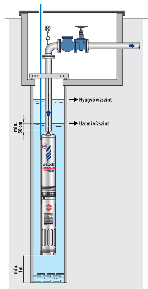
Tipikus telepítés
