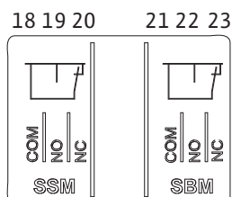
Fig. 15: Kapcsok SSM-hez és SBM-hez
