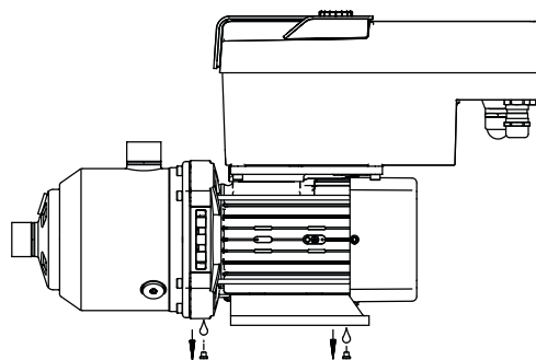
Fig. 6: Kondenzátumlefolyó nyílásokkal
