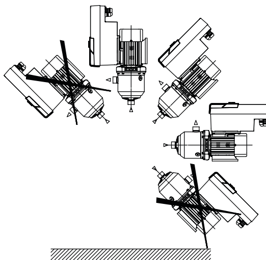
Fig. 5: A motortengely és felfelé néző elektronikamodul (0°) esetén megengedett beépítési helyzetek
