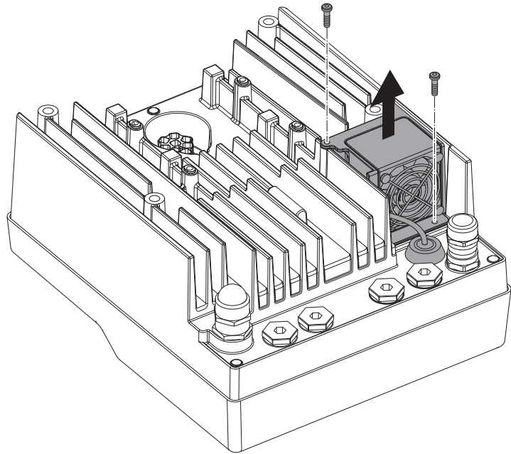
Fig. 47: A modulventilátor szétszerelése
