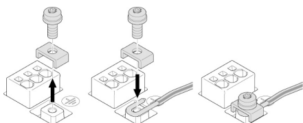
Fig. 14: Merev csatlakozókábel
