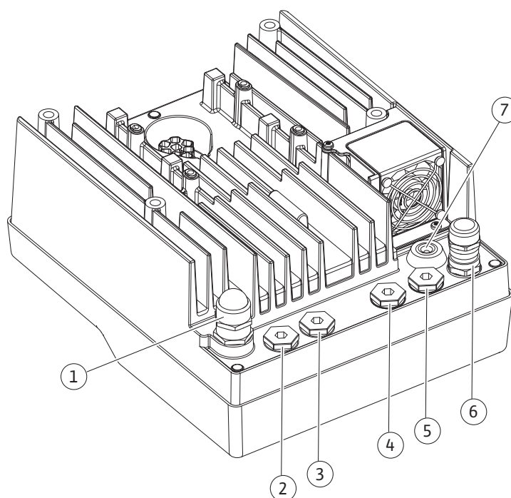
Fig. 10: Kábelcsavarzatok/Kábelcsatlakozások
