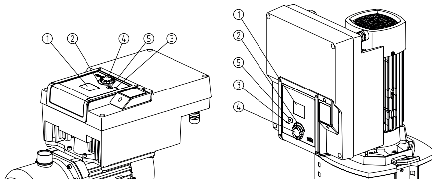
Fig. 19: Kezelőelemek
