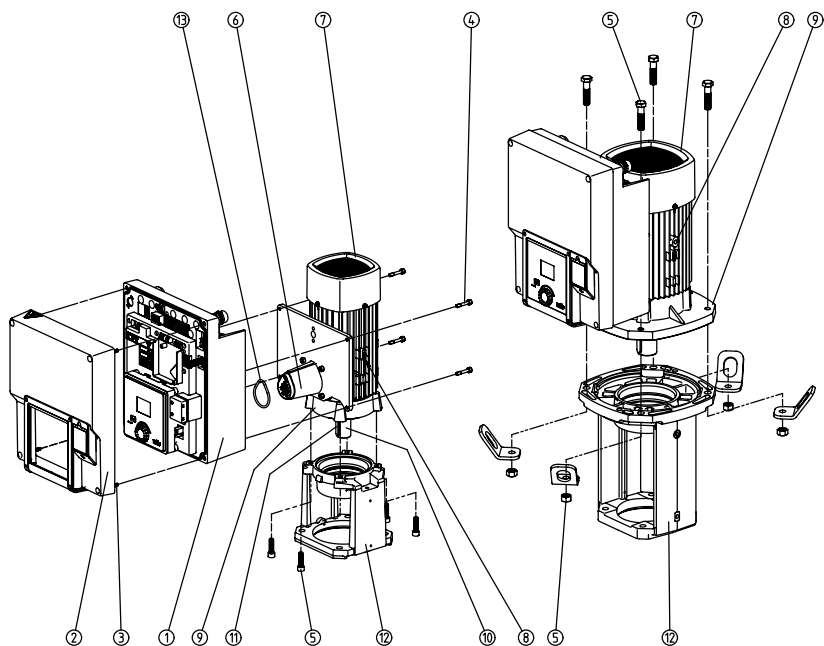
Fig. 1: Fő alkatrészek
