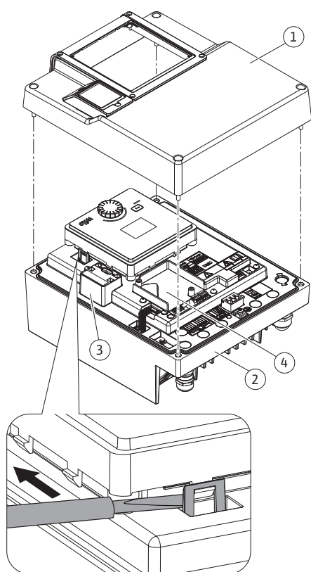
Fig. 17: Elektronikamodul
