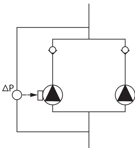
Fig. 9: Példa egy nyomáskülönbség-jeladó csatlakoztatására a közös gyűjtőcsőben.
